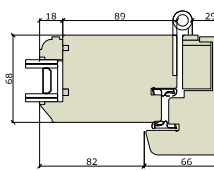
Jamb Section
